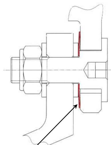
【断面図】
